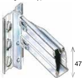
Longerons type S1/S2/S3
